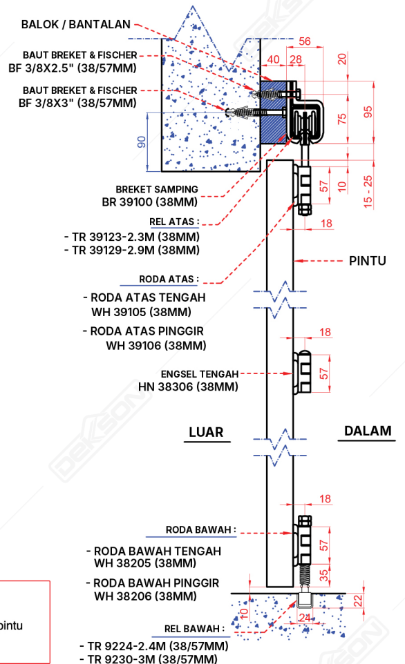
Gambar Potongan
