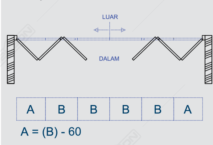
Gambar Tampak Atas
