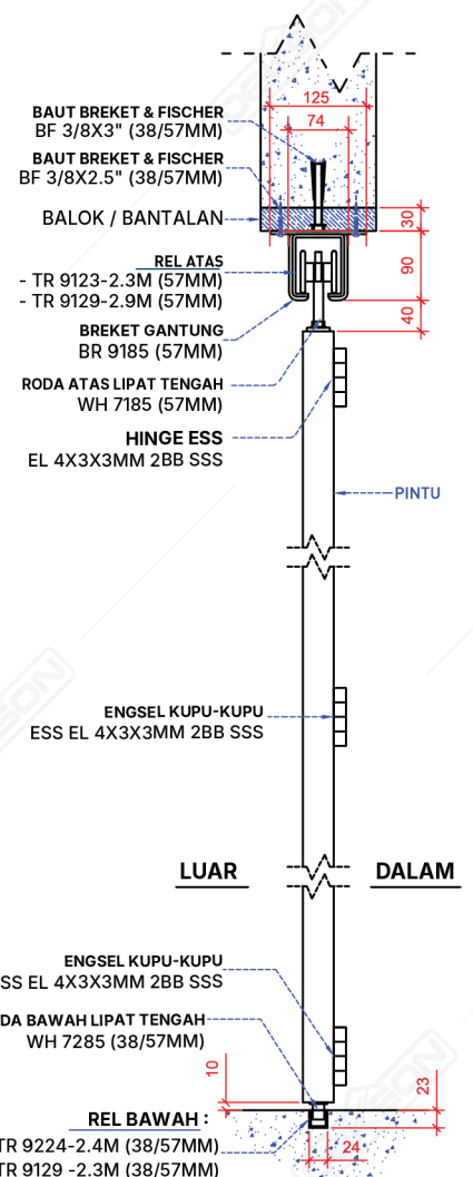
Gambar Potongan
