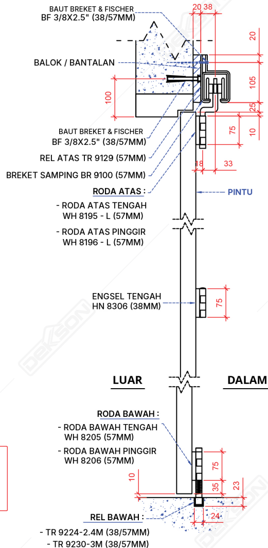
Gambar Potongan
