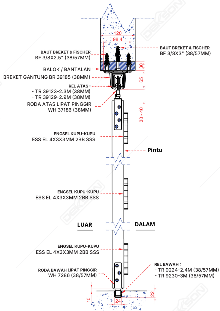
Gambar Potongan
