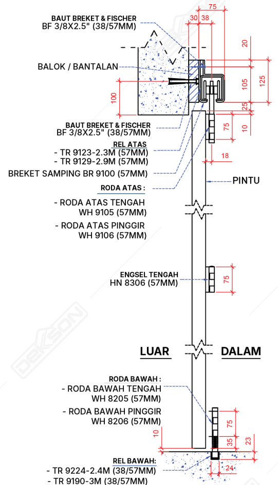
Gambar Potongan
