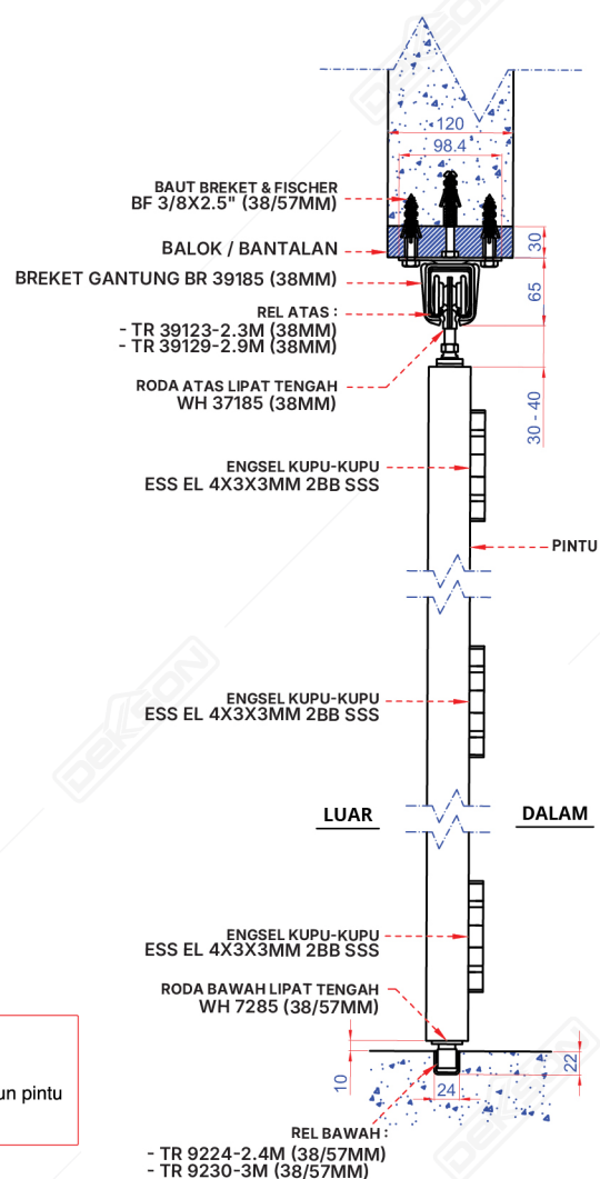
Gambar Potongan
